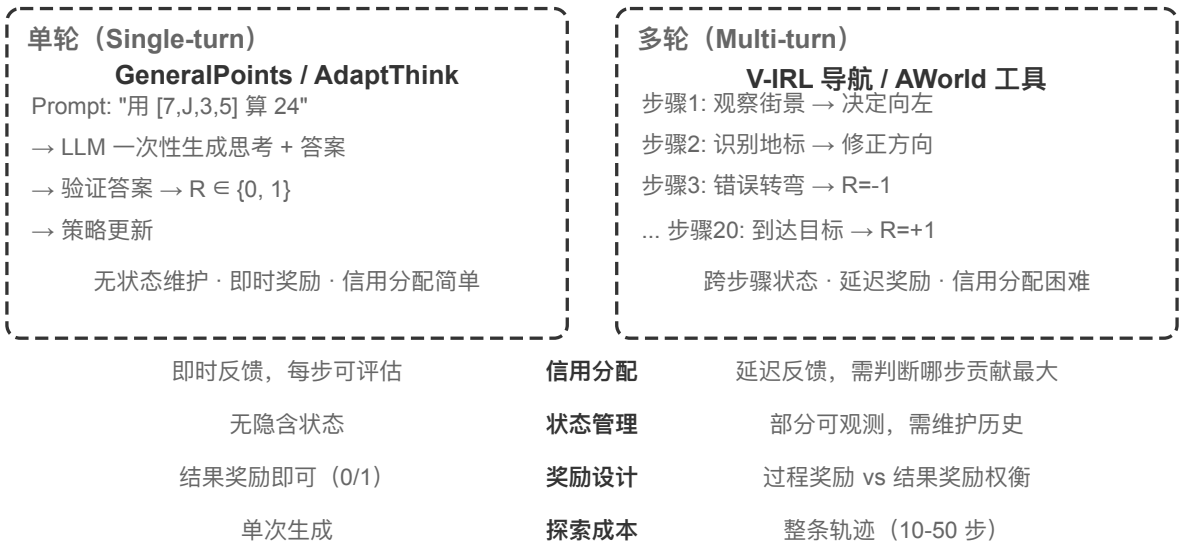
图 7-14 单轮 RL 与多轮 RL 对比
